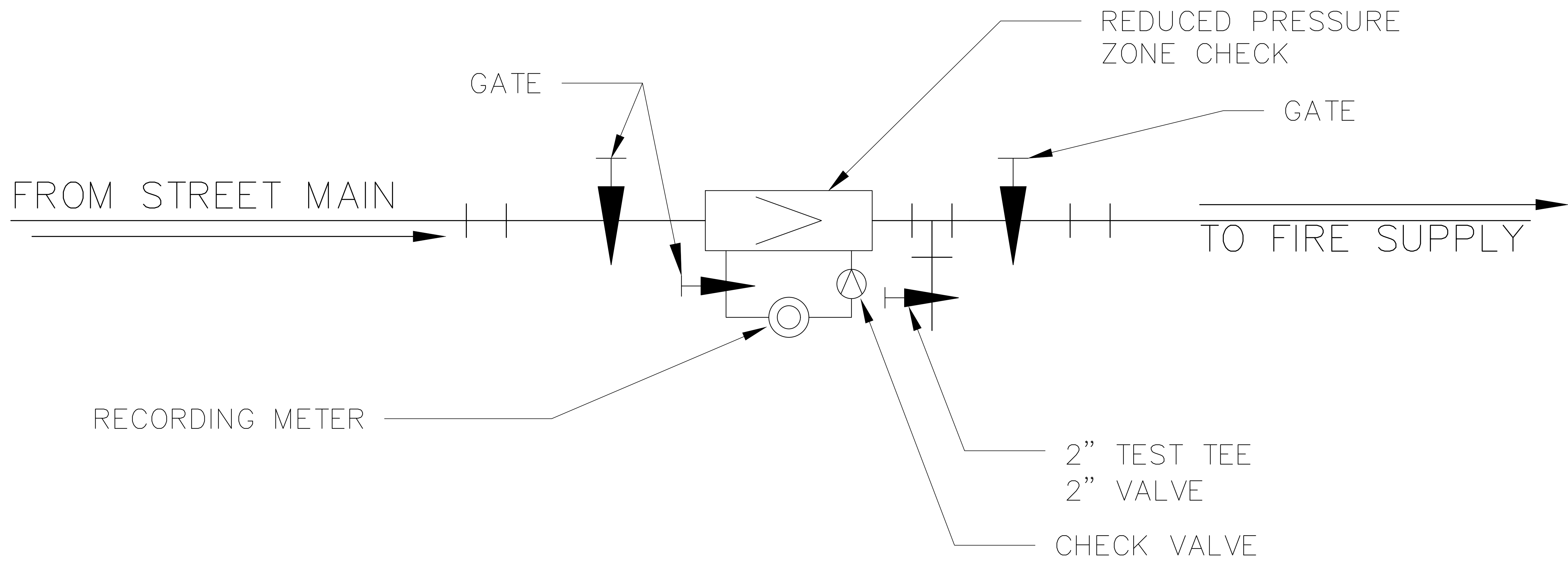
FIRE LINE METER SETTING DETAIL N.T.S.
